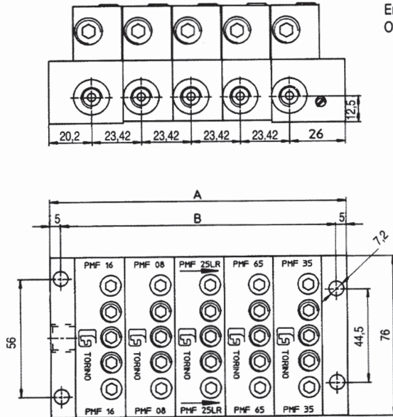
Dimensioni d'ingombro
